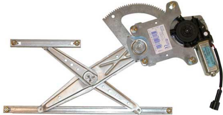
POWER WINDOW LEFT ALZACRISTALLI ELETTRICO SX
