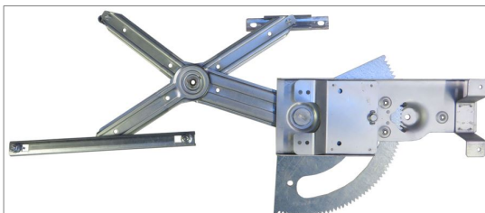
POWER WINDOW LEFT ALZACRISTALLI ELETTRICO SX
