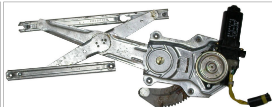
ORIGINAL POWER WINDOW LEFT ALZACRISTALLI ELETTRICO ORIGINALE SX
